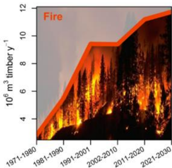
Danni da incendi forestali in milioni di metri cubi all'anno tra il 1971 ed oggi e previsione per il 2030 in Europa alla luce del cambiamento climatico in atto (fonte: Seidl et al. 2014, modificato)
