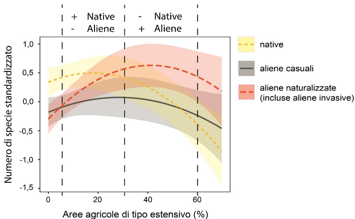
Andamento del numero cumulato di specie native, aliene casuali ed invasive in Friuli Venezia Giulia in relazione alla percentuale di paesaggio occupata da aree agricole di tipo estensivo.
